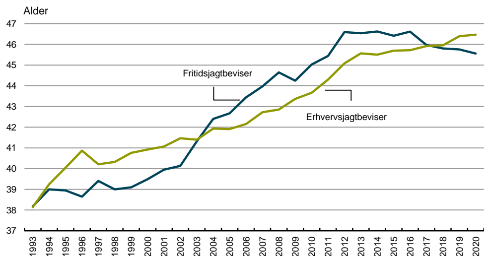
Figur 2. Udvikling af den gennemsnitlige alder fordelt på bevistype
